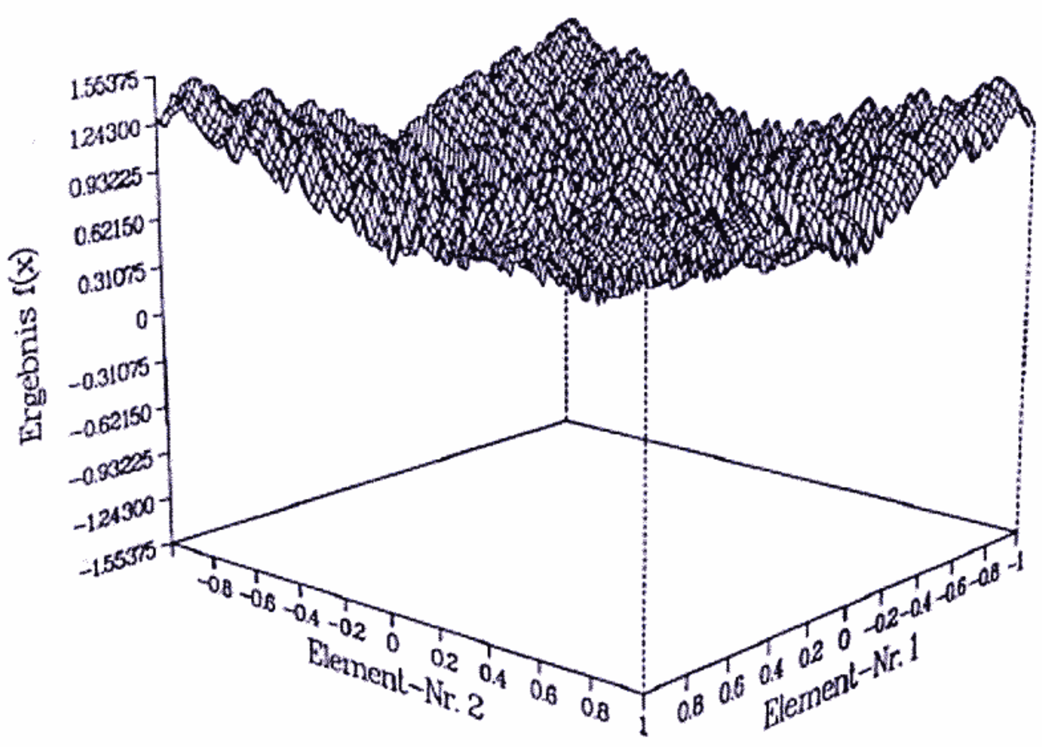
Testfunktion Nr. 88 f(x) Konstanten - keine
